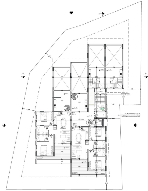
ΚΑΤΩΦΗ ΜΕΣΟΠΛΩΜΑΤΟΣ 1 ης ΟΡΟΦΟΥ
