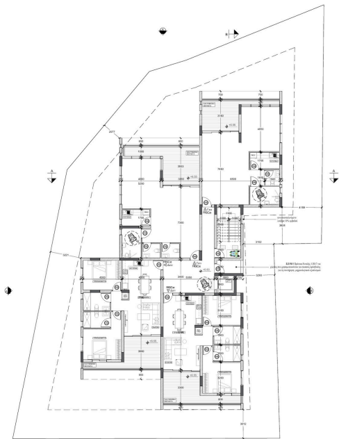
ΚΑΤΩΦΗ 2 ης ΟΡΟΦΟΥ
