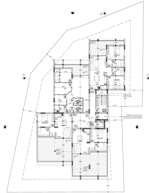
ΚΑΤΩΦΗ 3ης ΟΡΟΦΟΥ
