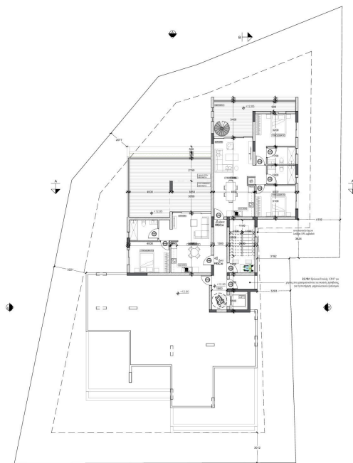
ΚΑΤΩΦΗ 4ης ΟΡΟΦΟΥ
