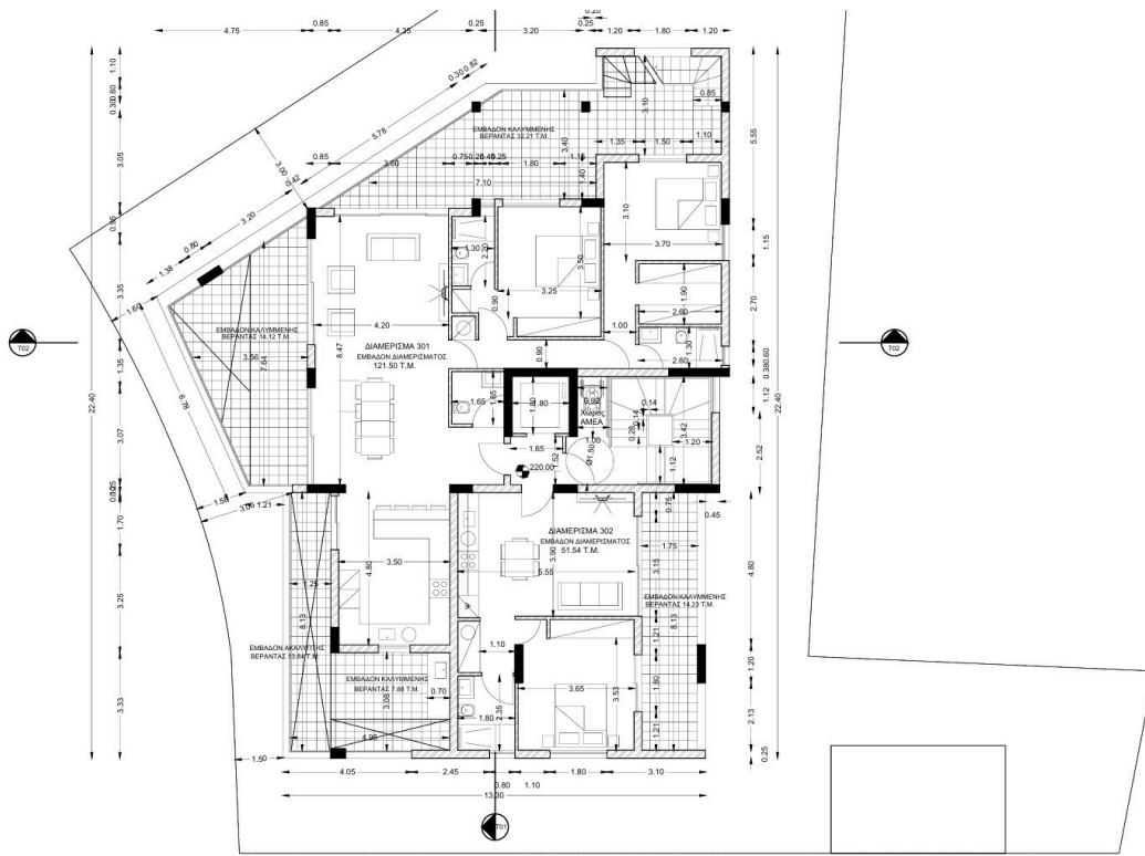
ΚΑΤΟΨΗ 3ΟΥ ΟΡΟΦΟΥ 1-100
