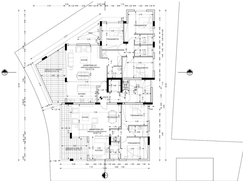
ΚΑΤΟΨΗ 2ΟΥ ΟΡΟΦΟΥ 1-100
