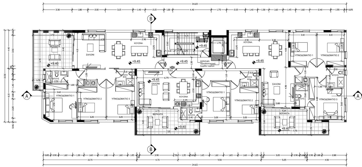
ΚΑΤΟΨΗ 3ου ΟΡΟΦΟΥ ΚΛΙΜΑΚΑ 1:100
