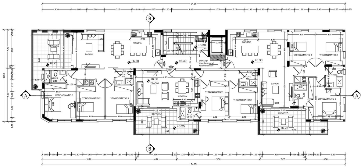
ΚΑΤΟΨΗ 2ου ΟΡΟΦΟΥ ΚΛΙΜΑΚΑ 1:100
