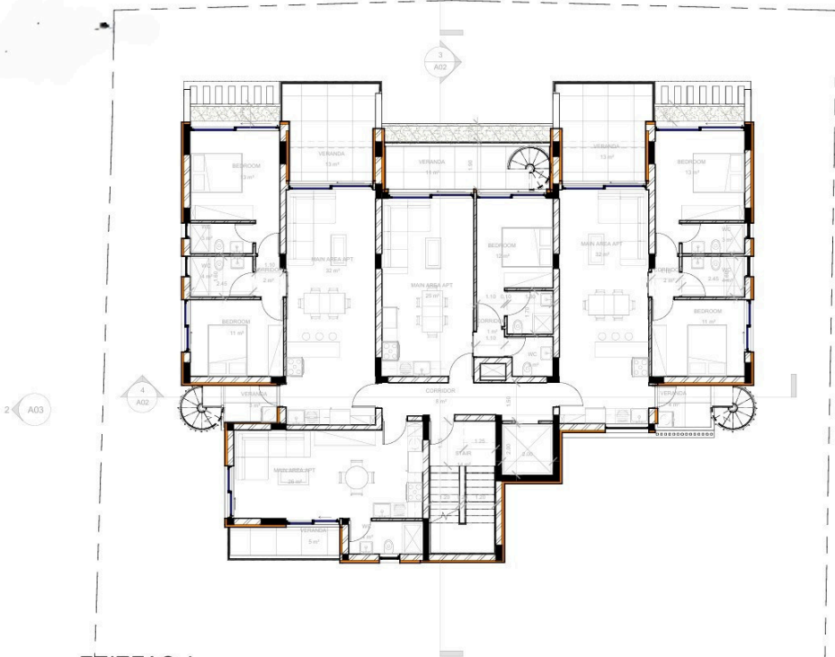
4 ΕΠΙΠΕΔΟ 4 1 : 100
