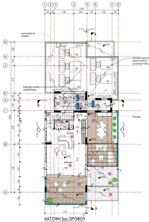
ΚΑΤΩΦΗ 3ου ΟΡΟΦΟΥ
