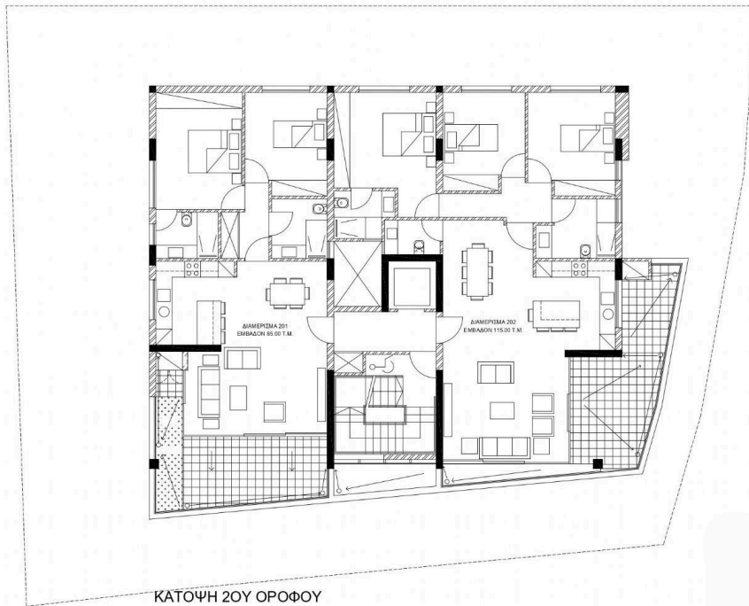
ΚΑΤΟΨΗ 2ΟΥ ΟΡΟΦΟΥ
