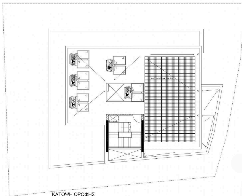
ΚΑΤΟΨΗ ΟΡΟΦΗΣ
