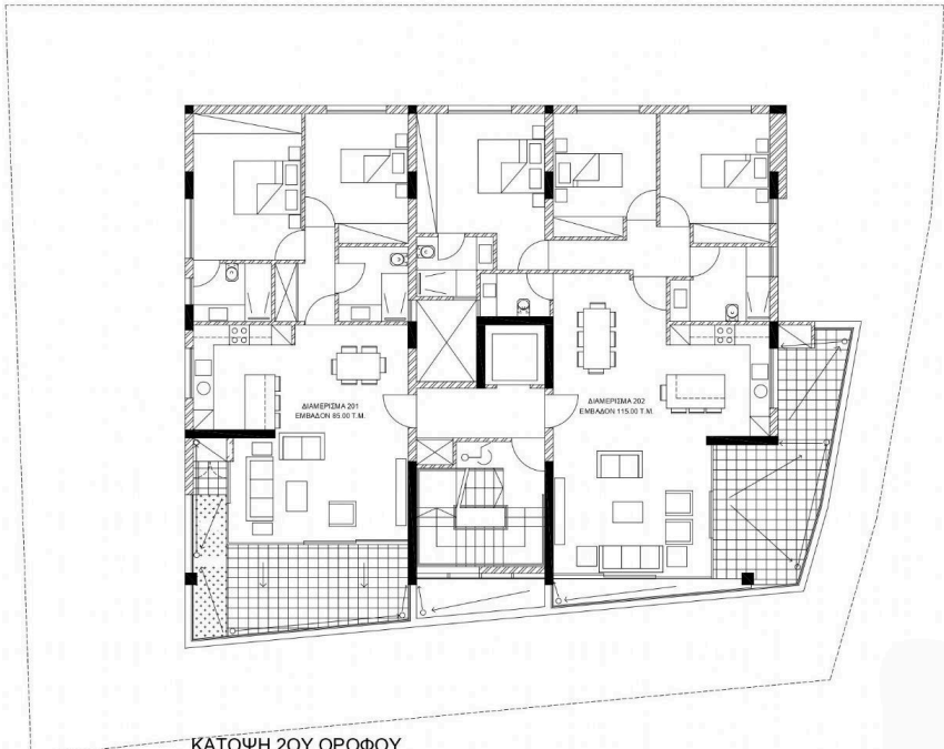
ΚΑΤΟΨΗ 2ΟΥ ΟΡΟΦΟΥ
