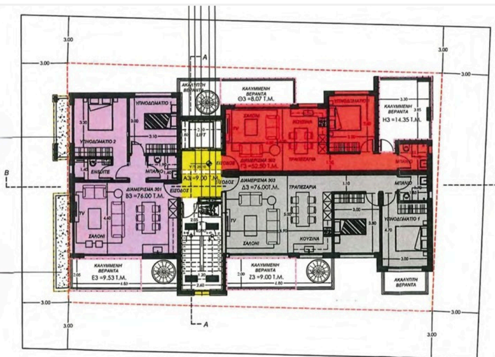
ΚΑΤΟΨΗ 3ου ΟΡΟΦΟΥ κλίμακα 1/200
