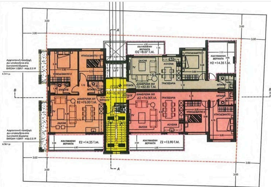
ΚΑΤΟΨΗ 2ου ΟΡΟΦΟΥ κλίμακα 1/200
