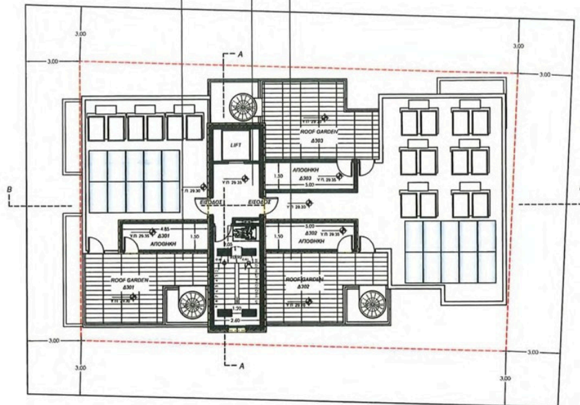
ΚΑΤΟΨΗ ΟΡΟΦΗΣ - ROOF GARDEN κλίμακα 1/200
