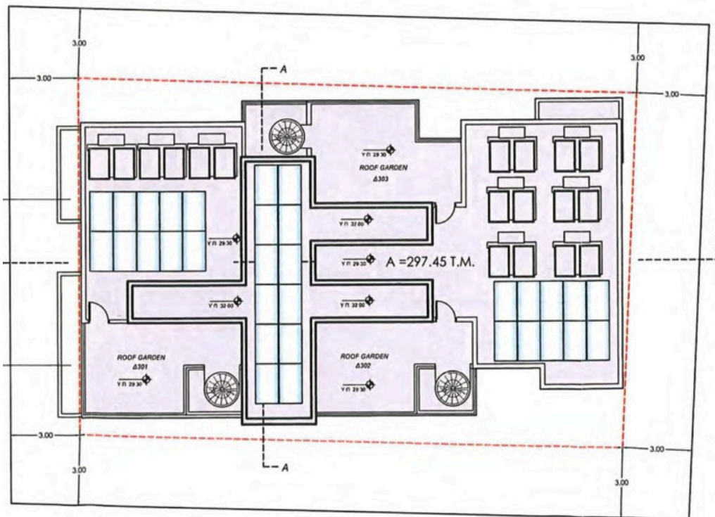
ΚΑΤΟΨΗ ΔΩΜΑΤΟΣ κλίμακα 1/200
