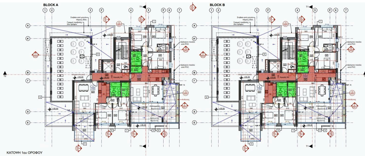
ΚΑΤΟΨΗ 1ου ΟΡΟΦΟΥ
