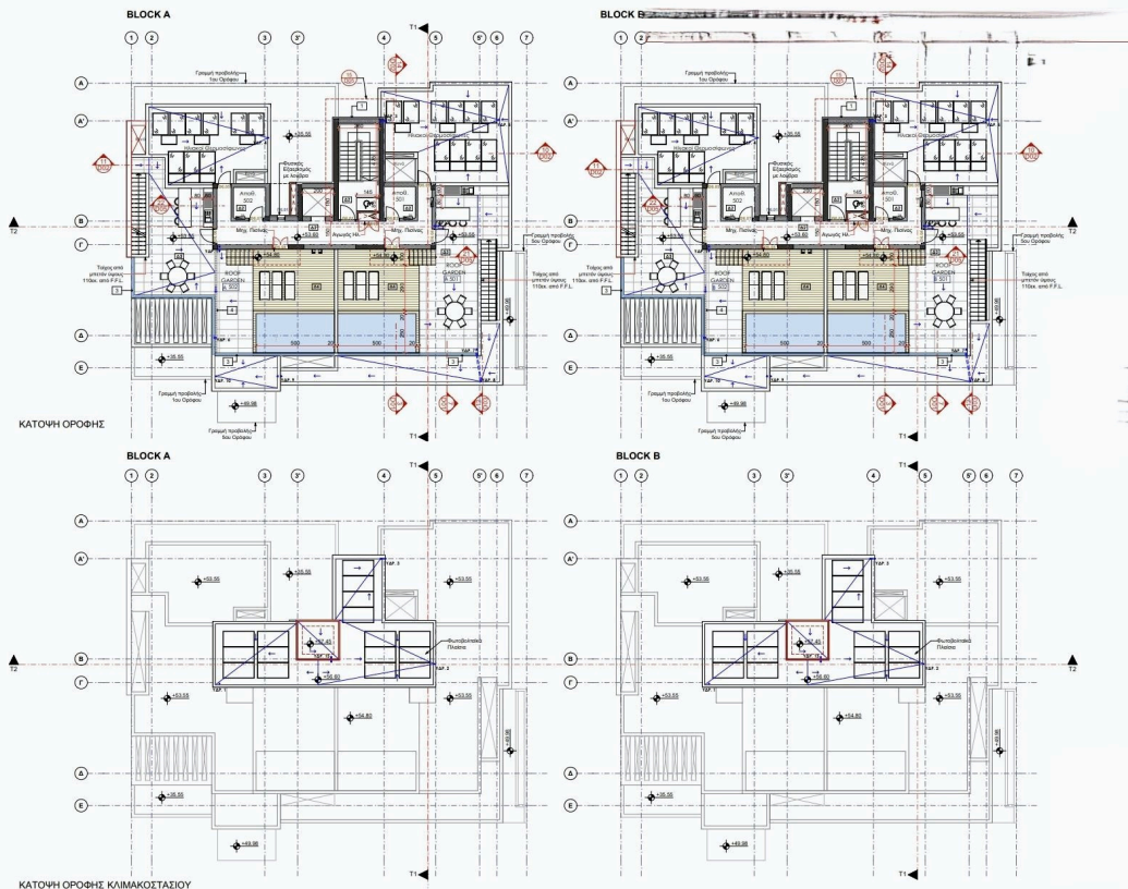
ΚΑΤΟΥΗ ΟΡΟΦΗΣ ΚΛΙΜΑΚΟΣΤΑΣΙΟΥ
