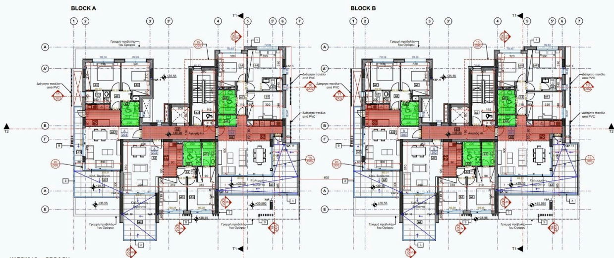
ΚΑΤΟΨΗ 2ου ΟΡΟΦΟΥ
