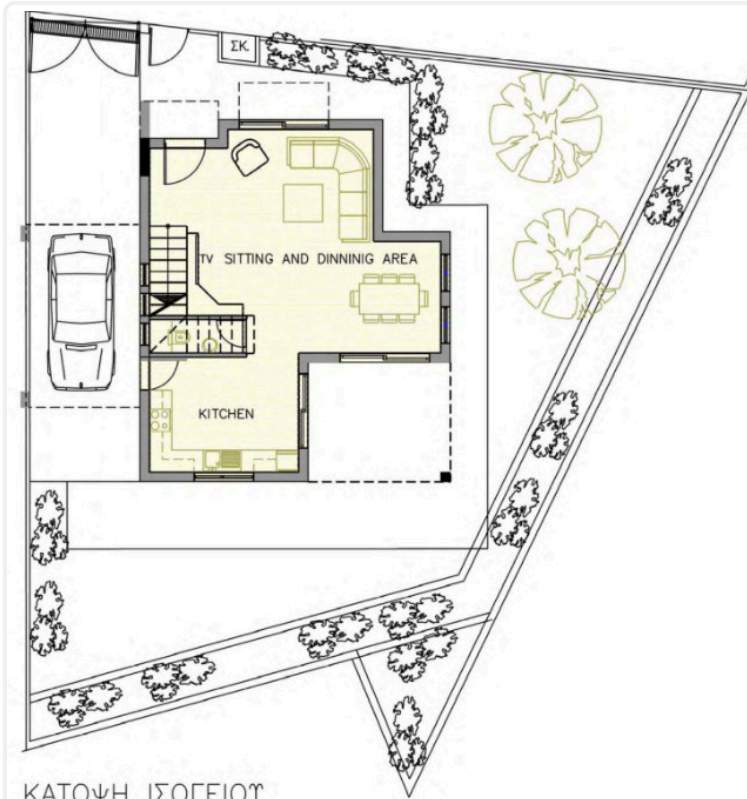
ΚΑΤΟΨΗ ΙΣΟΓΕΙΟΥ HOUSE 3
