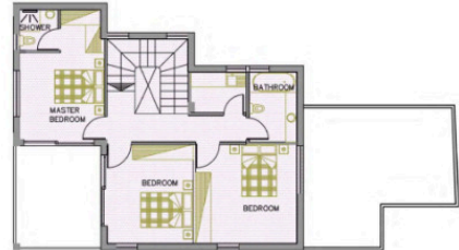
ΚΑΤΩΦΗ ΟΡΟΦΟΥ HOUSE 2
