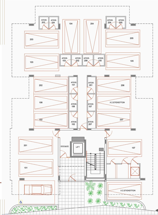
Κάτοψη Ισογείου
