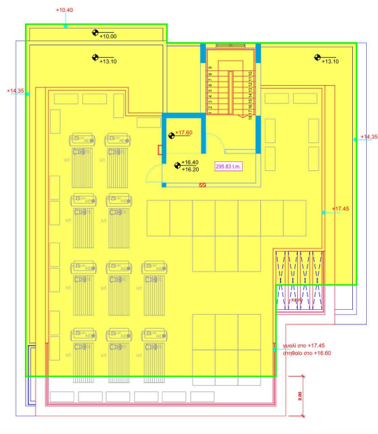
ΚΑΤΩΦΗ ΟΡΟΦΗΣ
