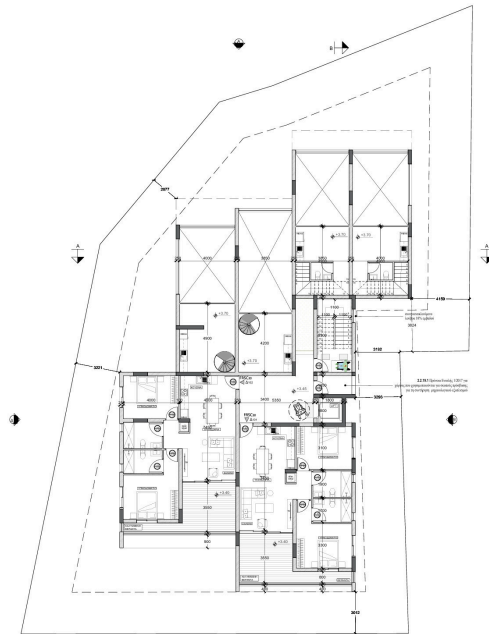
ΚΑΤΩΦΗ ΜΕΣΟΠΛΑΤΩΜΑΤΟΣ 1ου ΟΡΟΦΟΥ
