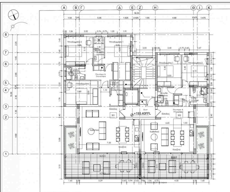
ΚΑΤΟΨΗ 3ΟΥ ΟΡΟΦΟΥ 1:100@A3
