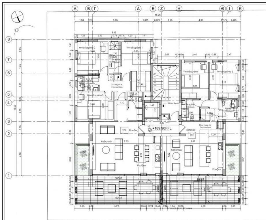
ΚΑΤΟΨΗ 2ΟΥ ΟΡΟΦΟΥ 1:100@A3
