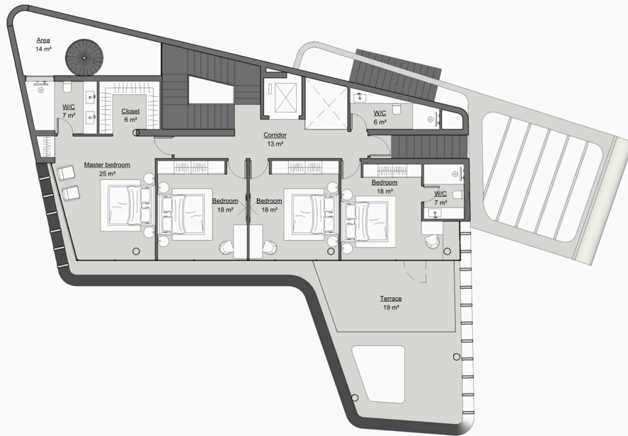
1 B1 Level 3 1 : 100
