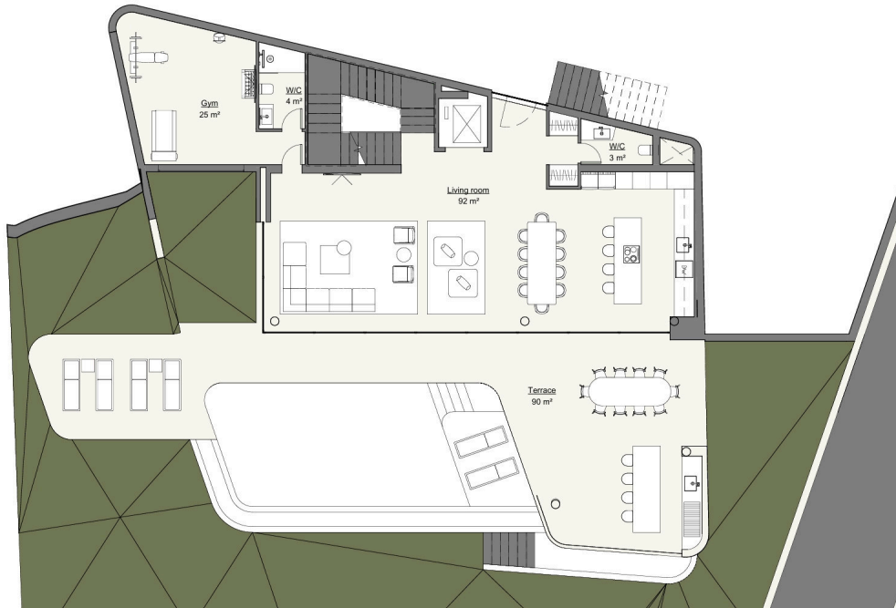
1 B1 Level 2 1 : 100
