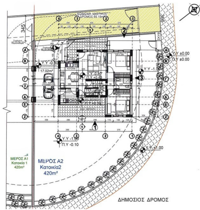
ΧΩΡΟΤΑΞΙΚΟ - ΚΑΤΩΝΗ ΙΣΟΓΕΙΟΥ ΚΛ. 1:200
