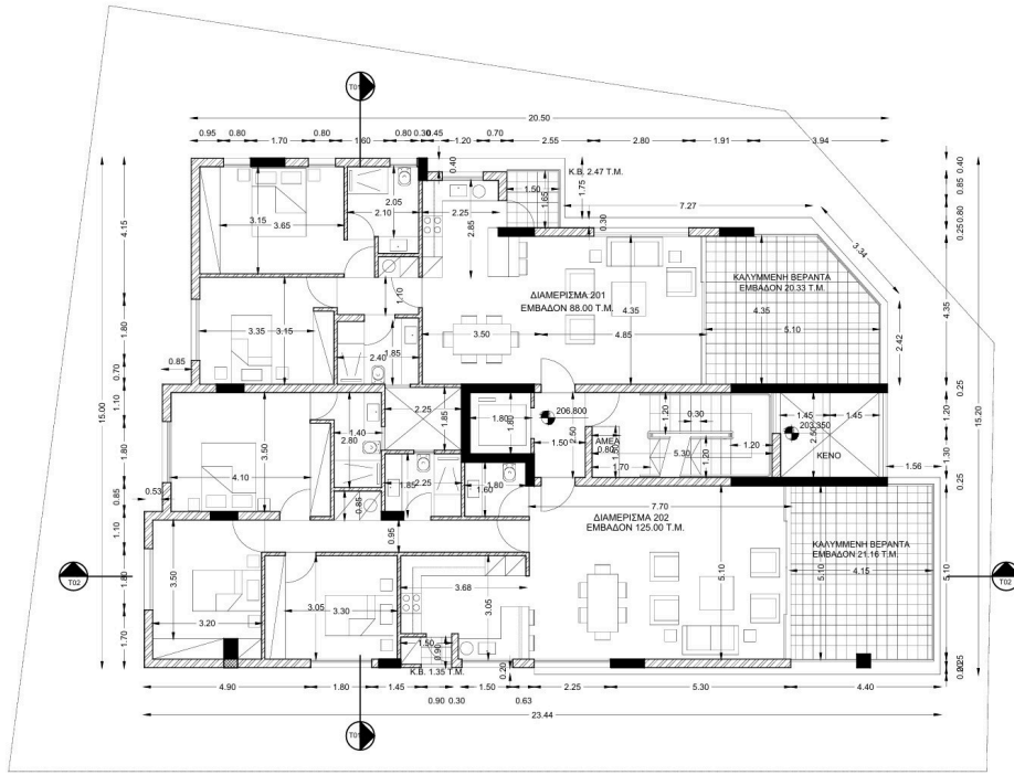
ΚΑΤΟΨΗ 2ΟΥ ΟΡΟΦΟΥ 1-100
