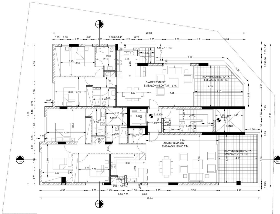
ΚΑΤΟΨΗ 3ΟΥ ΟΡΟΦΟΥ 1-100
