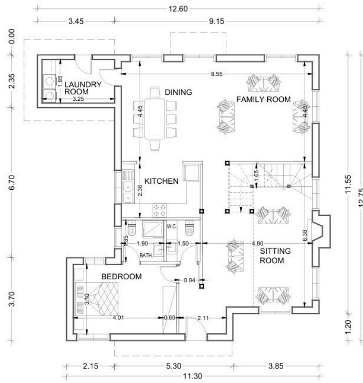
ΚΑΤΟΨΗ ΙΣΟΓΕΙΟΥ
