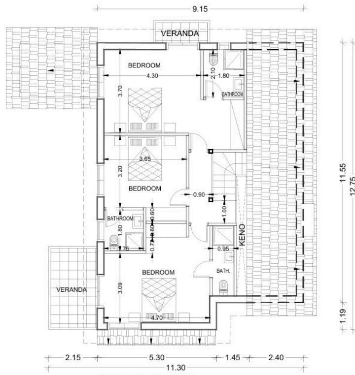
ΚΑΤΟΨΗ ΟΡΟΦΟΥ
