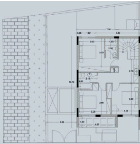
ΚΑΤΟΨΗ ΟΡΟΦΟΥ
