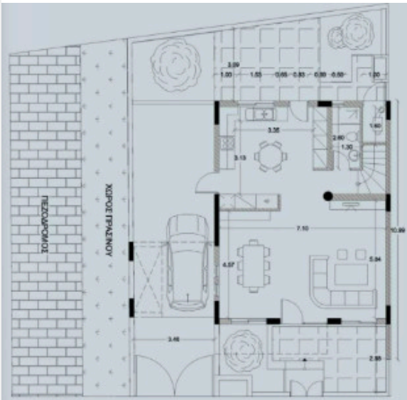
ΚΑΤΟΨΗ ΙΣΟΓΕΙΟΥ
