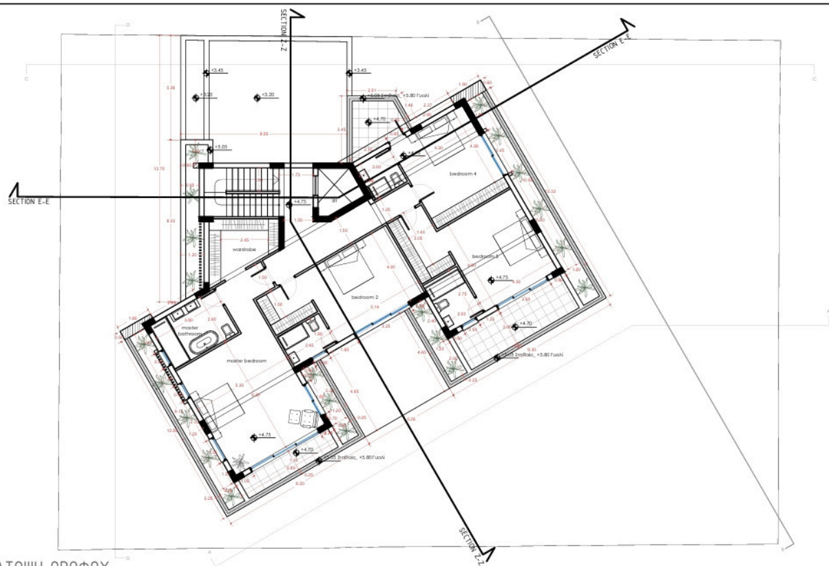
ΚΑΤΩΦΗ ΟΡΟΦΟΥ
