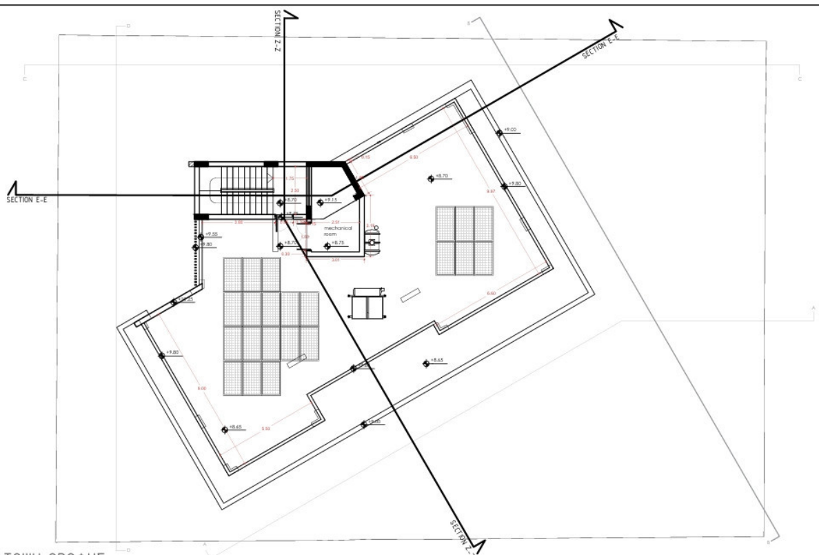
ΚΑΤΩΦΗ ΟΡΟΦΗΣ
