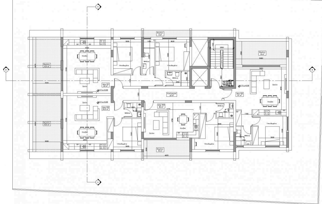
01 Κάτοψη 1ου ορόφου First floor plan
