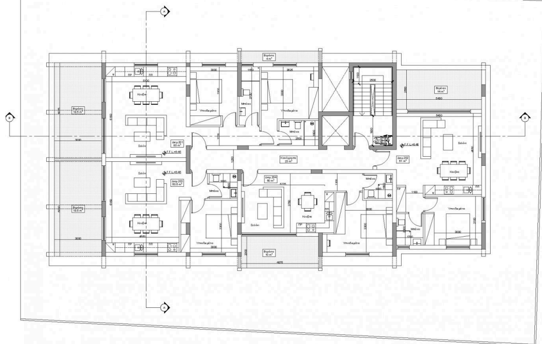
02 Κάτοψη 2ου ορόφου Second floor plan
