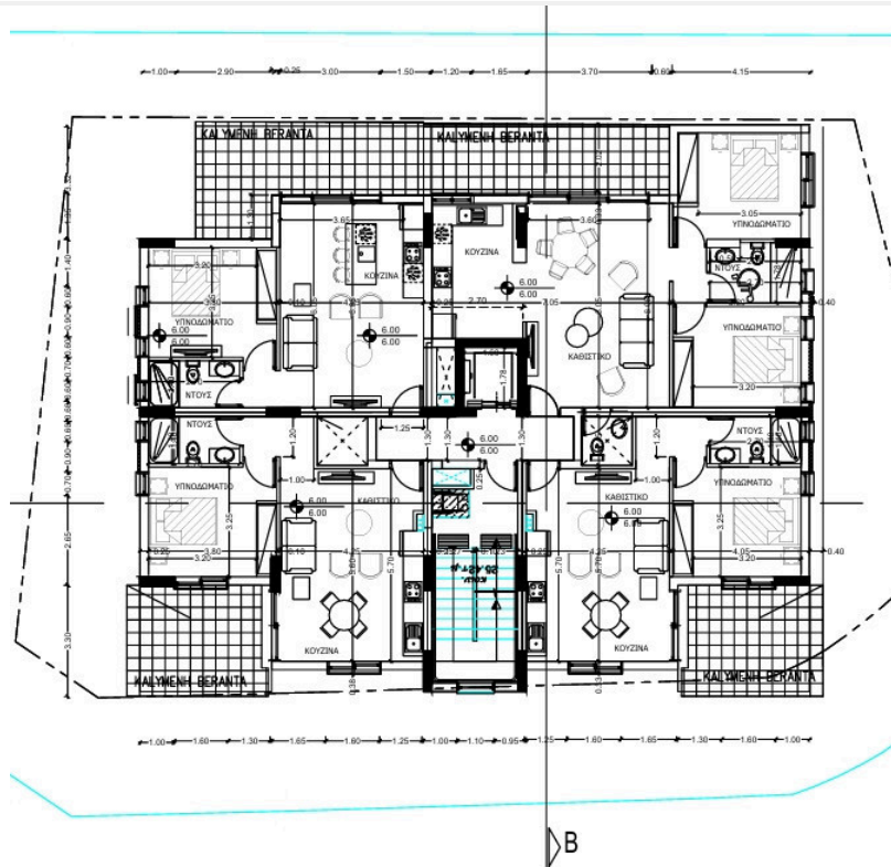
κατοψη δευτερου οροφου
