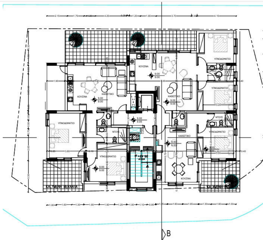
κατοψη τριτου οροφου
