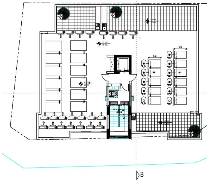
κατοψη οροφης
