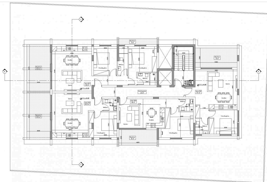
01 Κάτοψη 1ου ορόφου First floor plan
