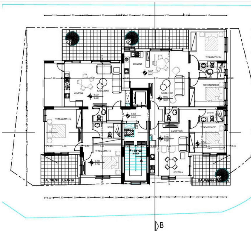
κατοψη τριτου οροφου
