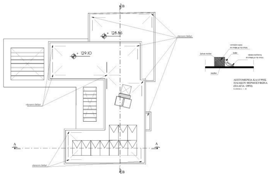
ΚΑΤΟΙΚΙΑ 2 ΚΑΤΟΨΗ ΟΡΟΦΗΣ ΚΛΙΜΑΚΑ 1:100
