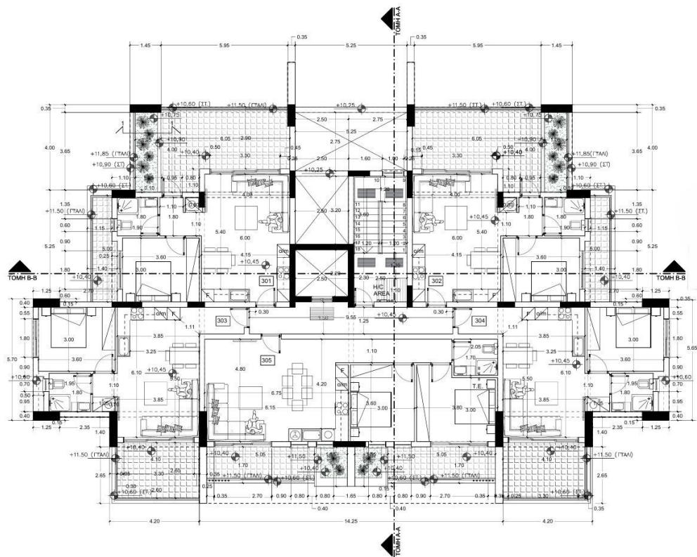
ΚΑΤΟΨΗ Γ ΟΡΟΦΟΥ
