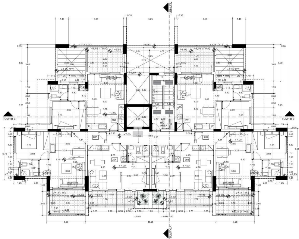
ΚΑΤΟΨΗ Β ΟΡΟΦΟΥ
