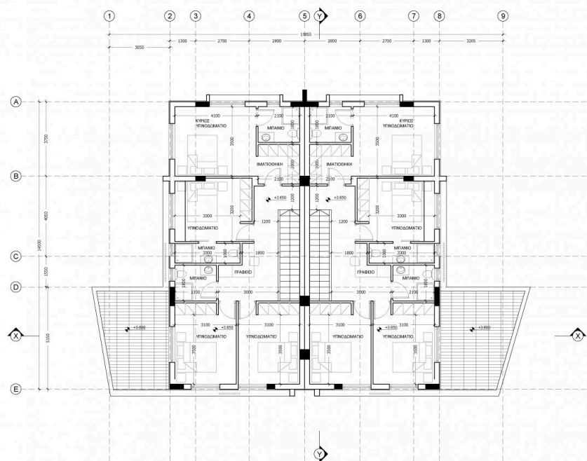
ΚΑΤΟΠΗ ΟΡΟΦΟΥ
