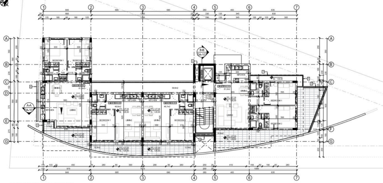
ΚΑΤΟΨΗ 2ου ΟΡΟΦΟΥ
