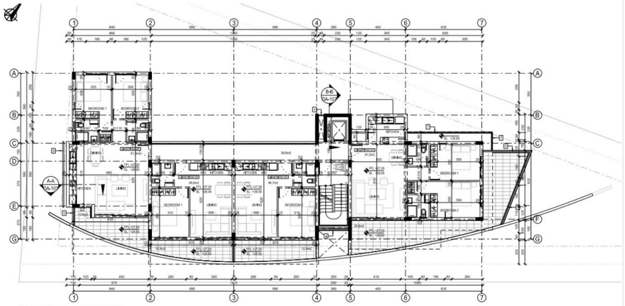
ΚΑΤΟΨΗ 2ου ΟΡΟΦΟΥ
