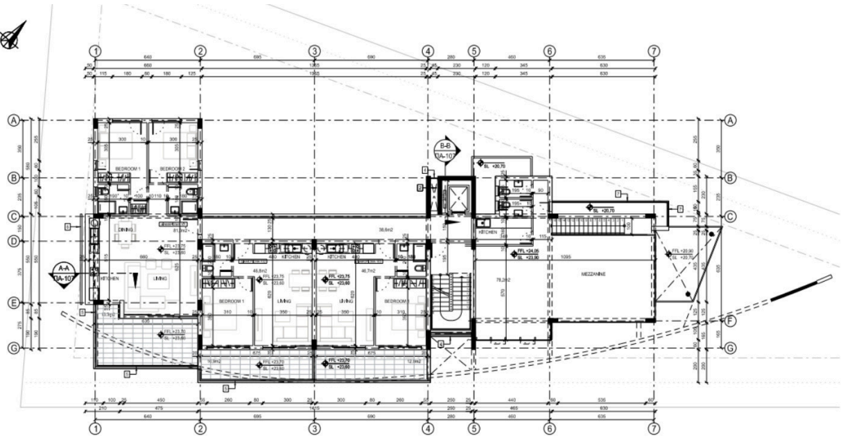
ΚΑΤΩΦΗ ΜΕΣΟΠΑΤΩΜΑΤΟΣ / 1ου ΟΡΟΦΟΥ
