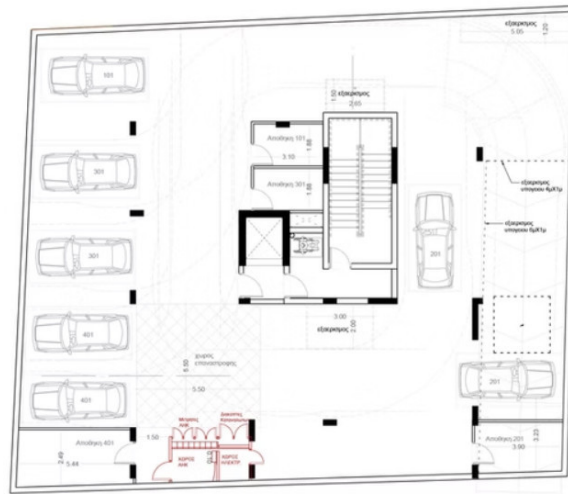
ΚΑΤΟΨΗ ΥΠΟΓΕΙΟΥ
