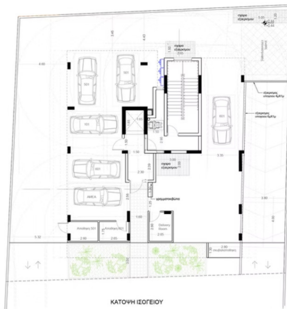
ΚΑΤΟΨΗ ΙΣΟΓΕΙΟΥ
