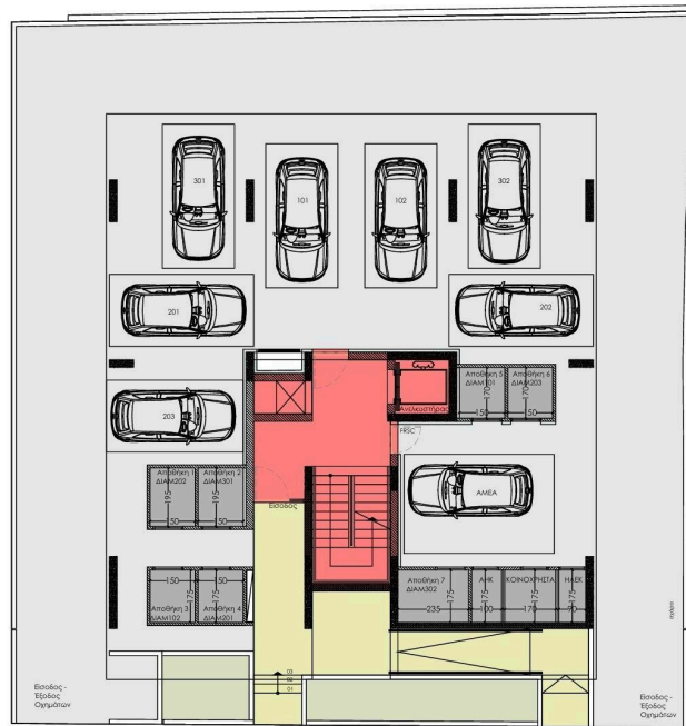
Κάτοψη Ισογείου
