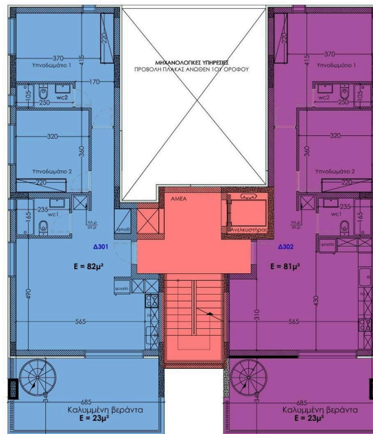
Κάτοψη 3ου ορόφου
