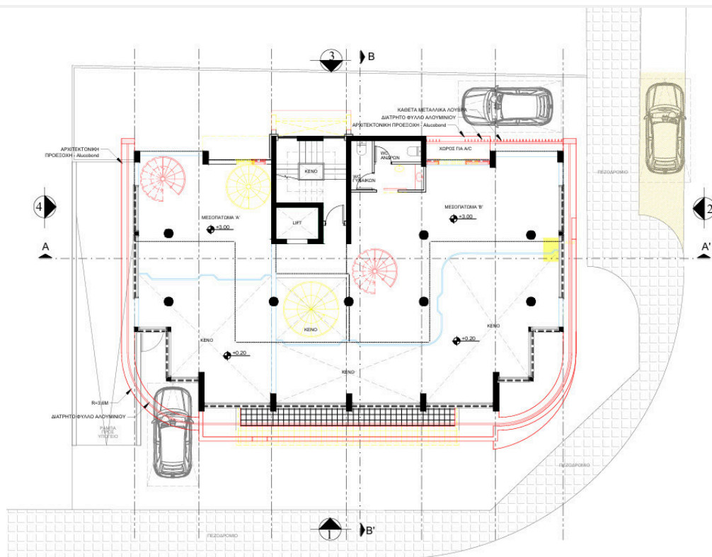
ΠΡΟΣΘΗΚΟΜΕΤΑΤΡΟΠΕΣ - ΚΑΤΟΨΗ ΜΕΣΟΠΑΤΩΜΑΤΟΣ Κλίμακα 1:100
