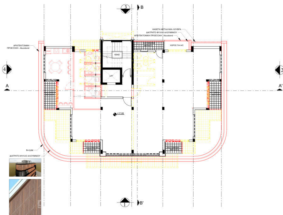
ΠΡΟΣΘΗΚΟΜΕΤΑΤΡΟΠΕΣ - ΚΑΤΟΨΗ 4ου ΟΡΟΦΟΥ Κλίμακα 1:100
