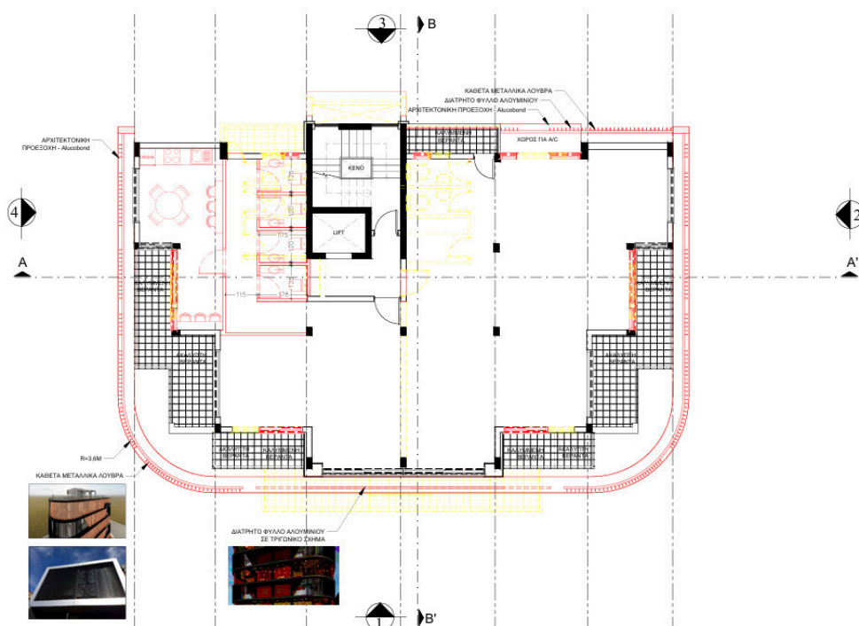
ΠΡΟΣΘΗΚΟΜΕΤΑΤΡΟΠΕΣ - ΚΑΤΟΨΗ 1ου ΟΡΟΦΟΥ Κλίμακα 1:100
