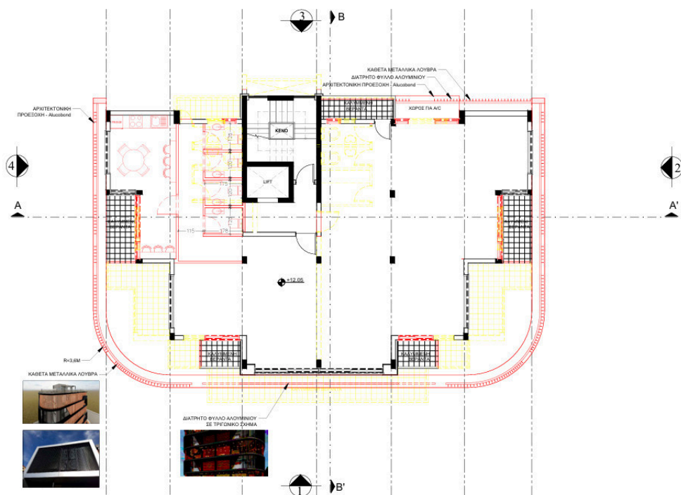
ΠΡΟΣΘΗΚΟΜΕΤΑΤΡΟΠΕΣ - ΚΑΤΟΨΗ 3ου ΟΡΟΦΟΥ Κλίμακα 1:100
