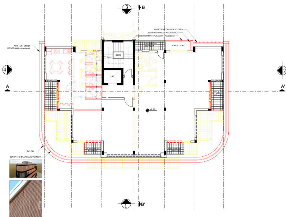
ΠΡΟΣΘΗΚΟΜΕΤΑΤΡΟΠΕΣ - ΚΑΤΟΨΗ 2ου ΟΡΟΦΟΥ Κλίμακα 1:100
