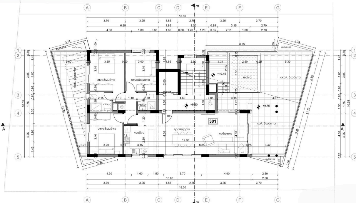
ΚΑΤΟΨΗ 3-ου ΟΡΟΦΟΥ 1:100
