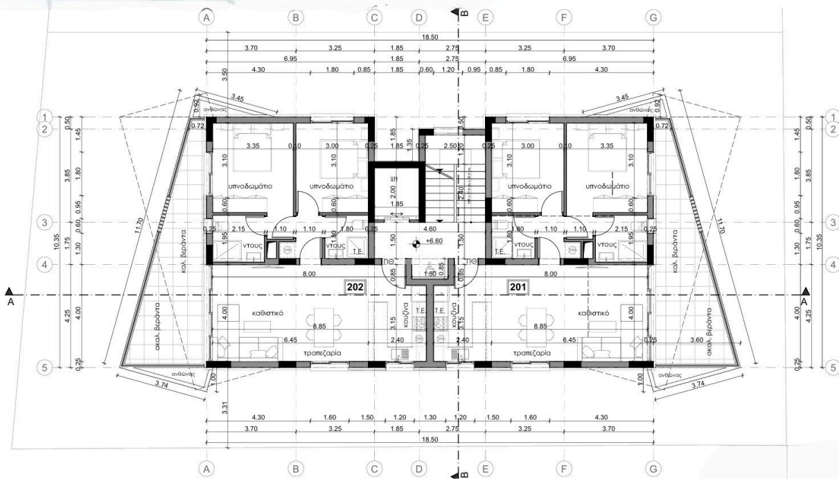
ΚΑΤΟΨΗ 2-ου ΟΡΟΦΟΥ 1:100
