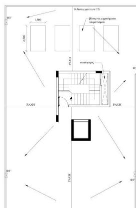
Κάτοψη ταράτσας
