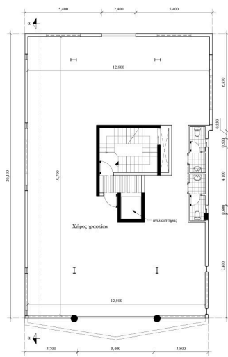
Κάτοψη τυπικού ορόφου (2ος & 3ος)
