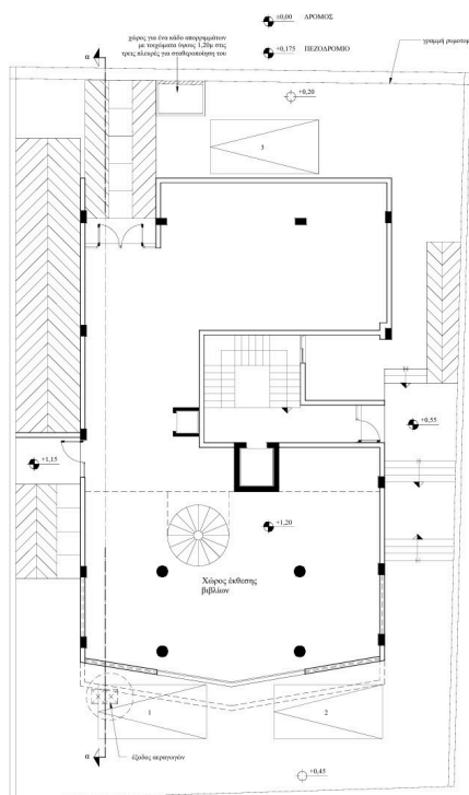
Κάτοψη ισογείου
