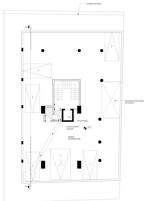
Κάτοψη υπογείου (-2)
