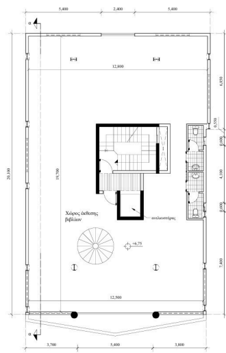
Κάτοψη 1ου ορόφου
