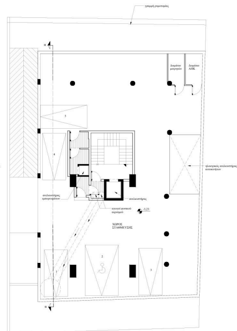
Κάτοψη υπογείου (-1)
