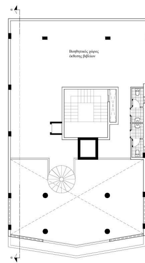
Κάτοψη μεσοπατώματος
