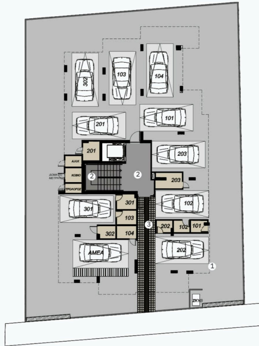
ΚΑΤΟΨΗ ΙΣΟΓΕΙΟΥ
