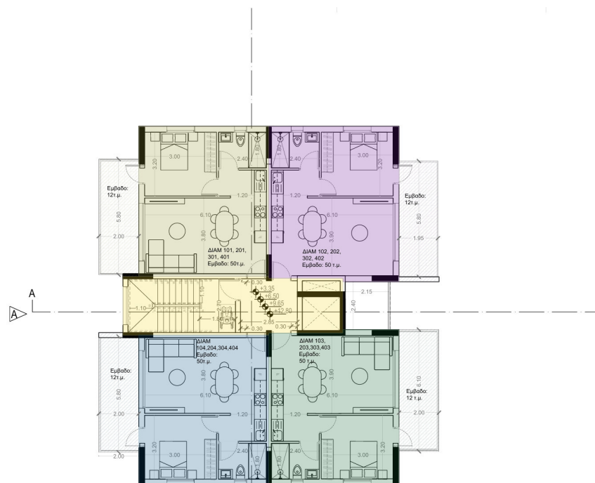
ΚΑΤΟΨΗ 1ΟΥ- 4ΟΥ ΟΡΟΦΟΥ
