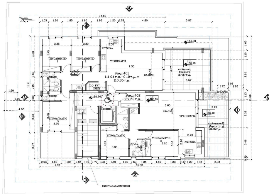
ΚΑΤΟΨΗ 4ου ΟΡΟΦΟΥ
