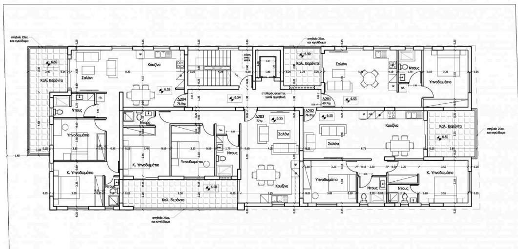
Κάτοψη 2ου Ορόφου
