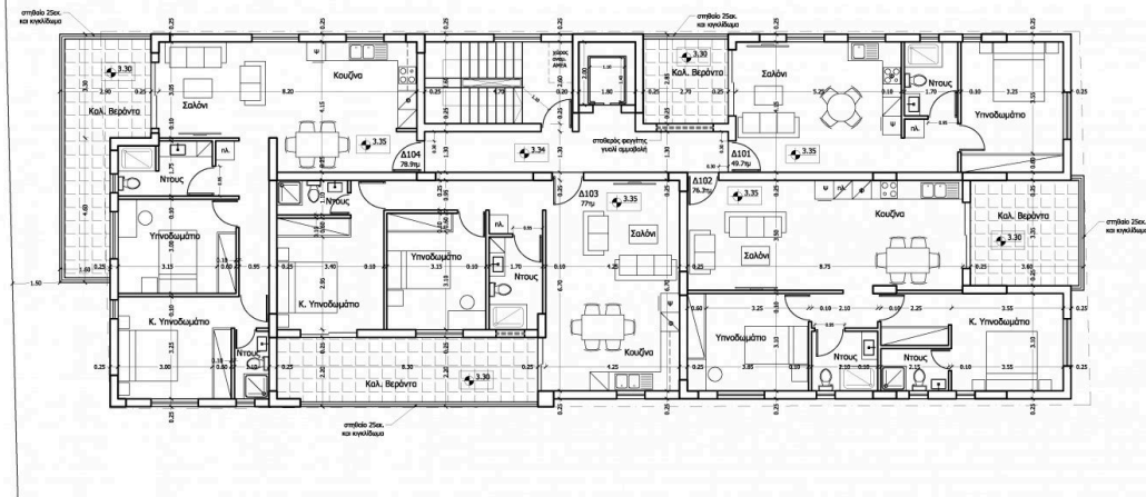
Κάτοψη 1ου Ορόφου
