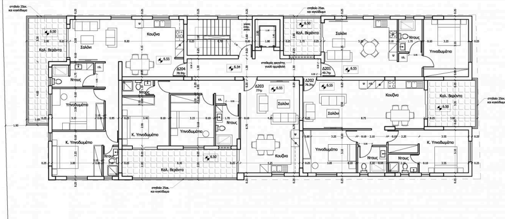
Κάτοψη 2ου Ορόφου
