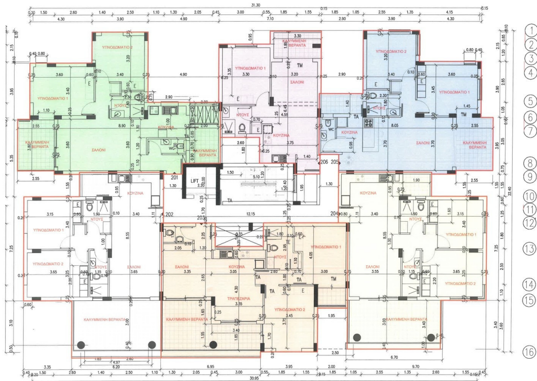
ΚΑΤΟΨΗ 2ου ΟΡΟΦΟΥ
