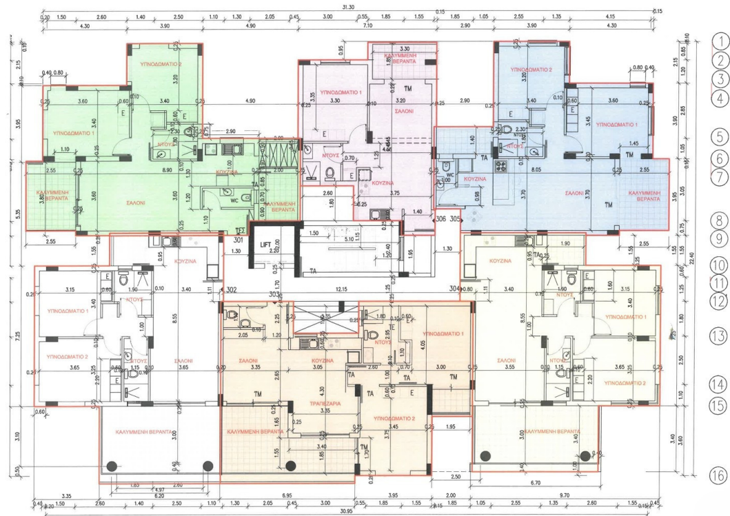
ΚΑΤΟΨΗ 3ου ΟΡΟΦΟΥ
