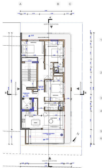
ΚΑΤΩΦΗ ΖΟΥ ΟΡΟΦΟΥ ΚΛΙΜΑΚΑ 1:200
