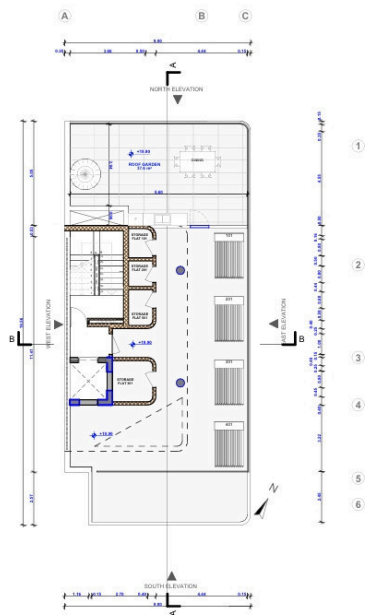
ΚΑΤΟΨΗ ROOF GARDEN ΚΛΙΜΑΚΑ 1:200
