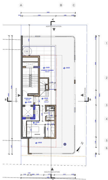
ΚΑΤΟΧΗ 5ΟΥ ΟΡΟΦΟΥ ΚΛΙΜΑΚΑ 1:200
