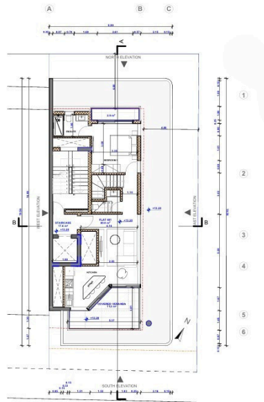
ΚΑΤΟΧΗ 4ΟΥ ΟΡΟΦΟΥ ΚΛΙΜΑΚΑ 1:200
