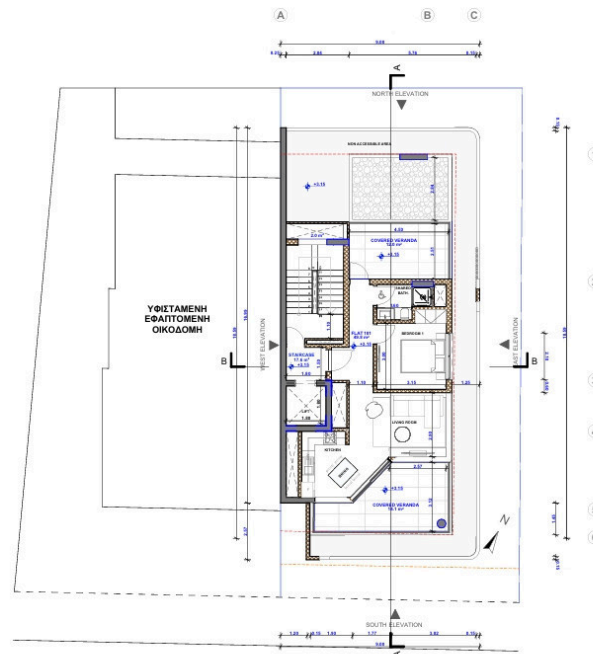
ΚΑΤΩΦΗ 1ΟΥ ΟΡΟΦΟΥ ΚΛΙΜΑΚΑ 1:200
