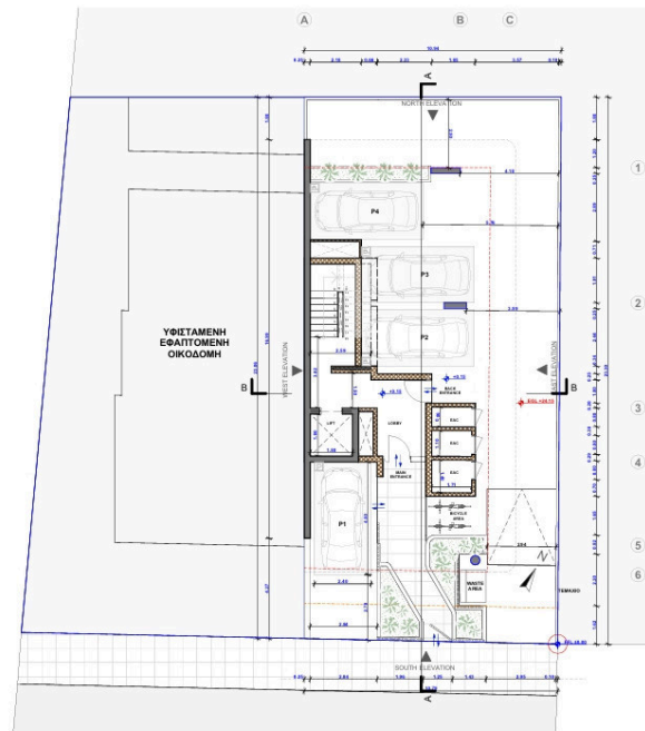
ΚΑΤΩΦΗ ΙΣΟΓΕΙΟΥ ΚΛΙΜΑΚΑ 1:200
