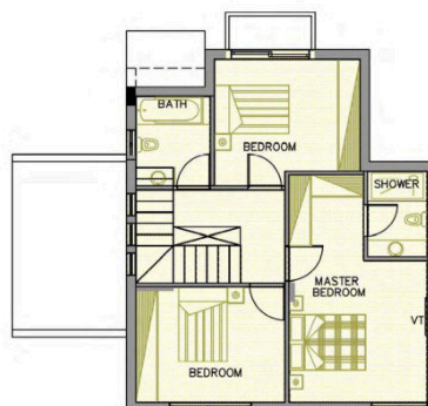
ΚΑΤΟΨΗ ΟΡΟΦΟΥ HOUSE 3
