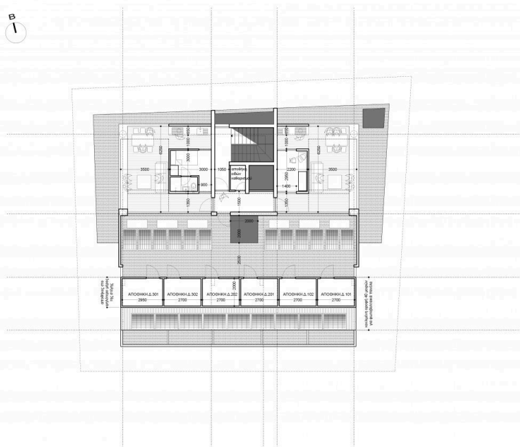
κάτοψη διώκτου_1:100
