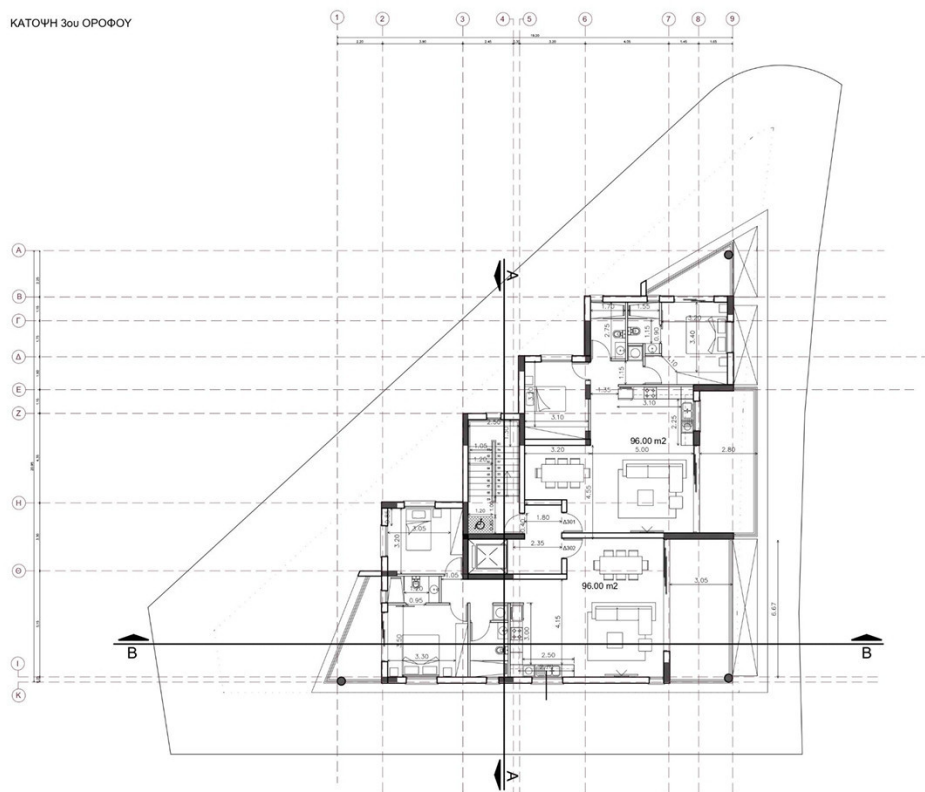
ΚΑΤΟΨΗ 3ου ΟΡΟΦΟΥ
