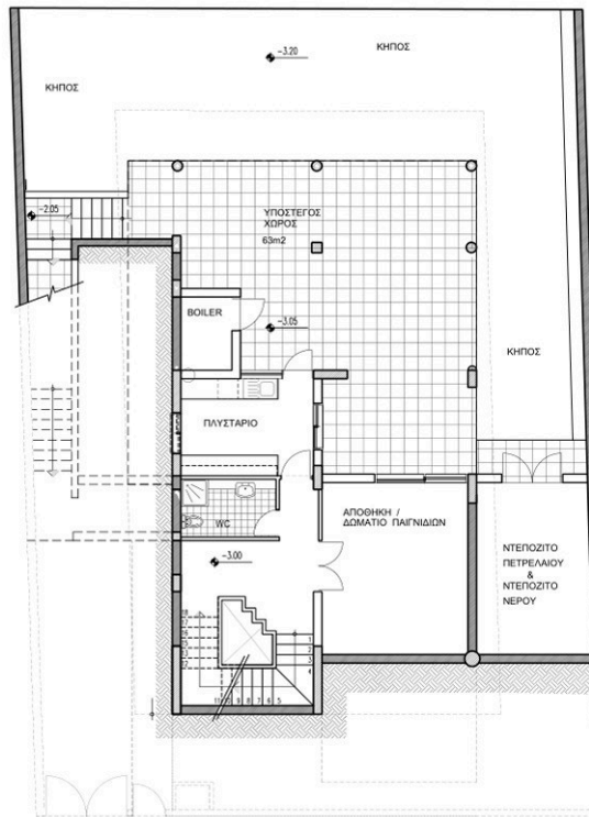
ΚΑΤΟΨΗ ΥΠΟΓΕΙΟΥ - 70m 2 & ΥΠΟΣΤΕΓΟΣ ΧΩΡΟΣ 63m 2
