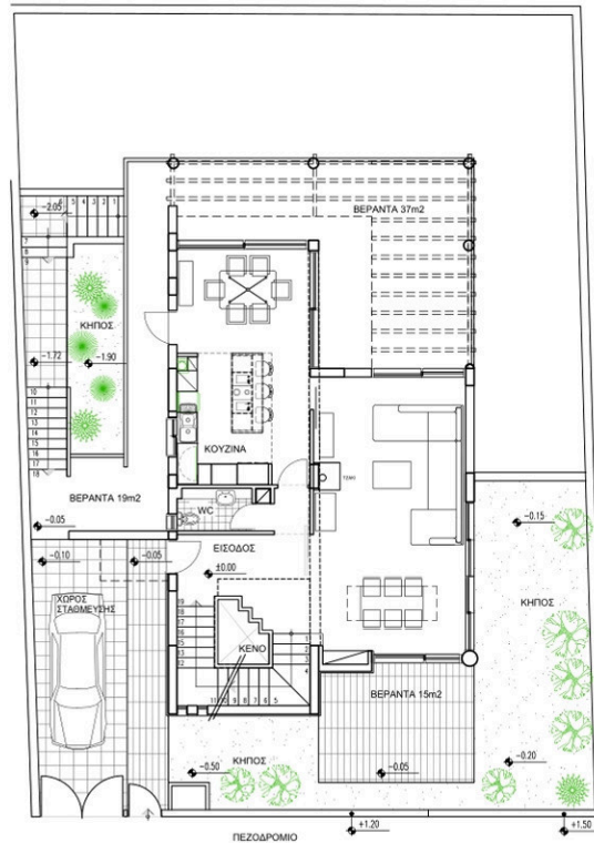
ΚΑΤΟΨΗ ΙΣΟΓΕΙΟΥ - 100m 2
