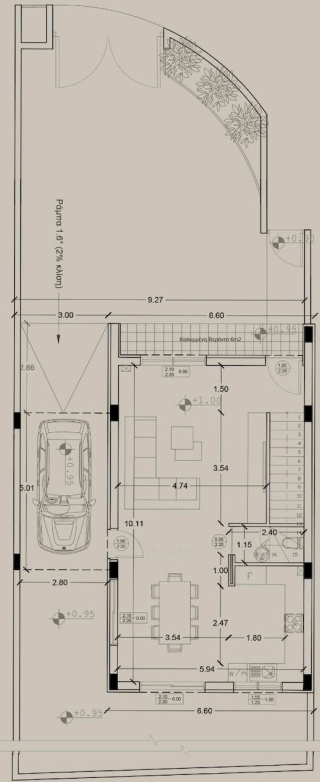
ΚΑΤΩΦΗ ΙΣΟΓΕΙΟΥ
