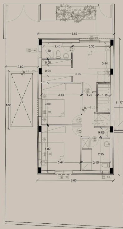
ΚΑΤΟΨΗ ΟΡΟΦΟΥ
