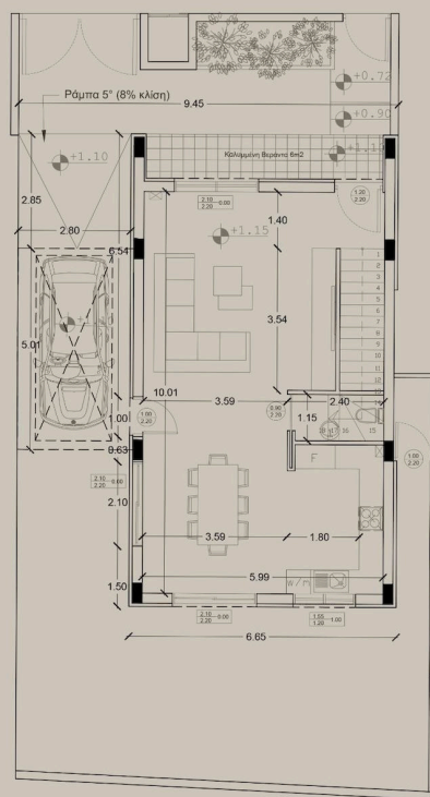
ΚΑΤΟΨΗ ΙΣΟΓΕΙΟΥ
