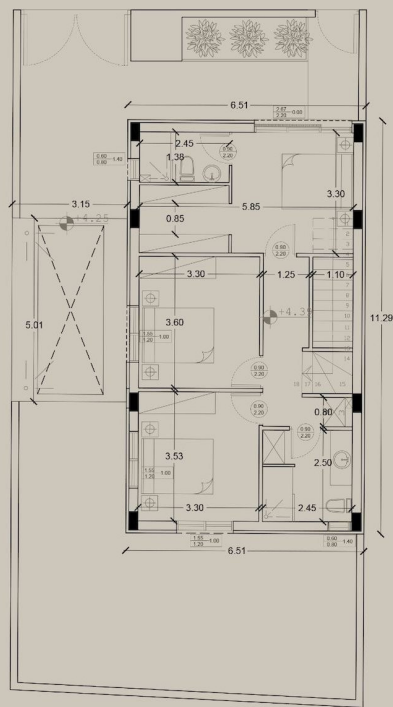
ΚΑΤΟΨΗ ΟΡΟΦΟΥ
