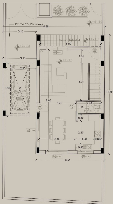
ΚΑΤΟΨΗ ΙΣΟΓΕΙΟΥ
